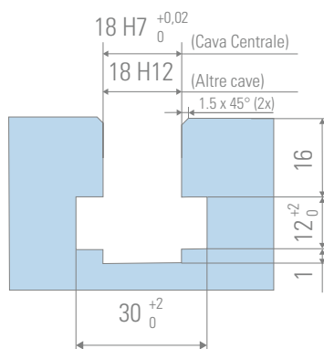
Sezione A-A
